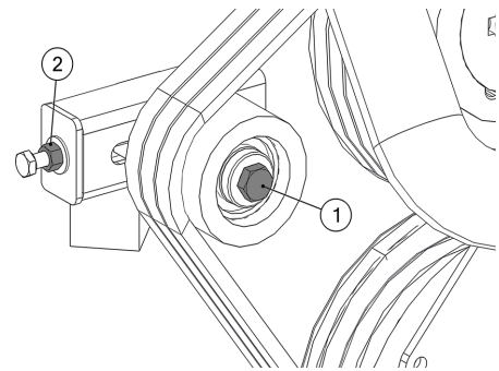
Afbeelding 22 - Poeliecomponent
