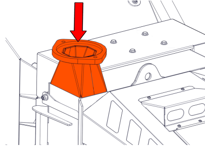
Afbeelding 27 - Uitwerpflezen - pijp verwijderd
