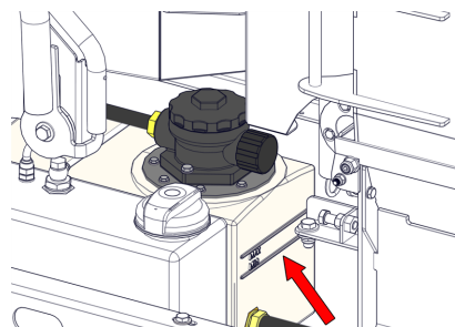
Afbeelding 17 - Indicator voor hydrauliekoliepeil
