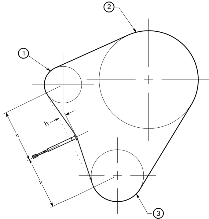
Afbeelding 24 - Schematisch overzicht van de rotoraandrijfriem
