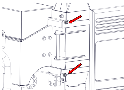
Afbeelding 19 - Toegangsklep motorbehuizing
