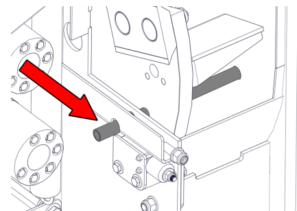
Afbeelding 20 - Grendelstang aangebracht
