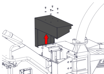
Afbeelding 28 - De beschermkap van de walskast verwijderen
