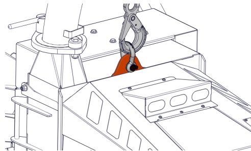
Afbeelding 18 - Hefoog en harpsluiting
