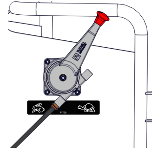
Afbeelding 9 - Gashendel
