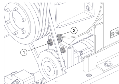
Afbeelding 23 - De pompriem afstellen
