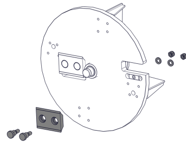
Afbeelding 21 - Montage van messen
