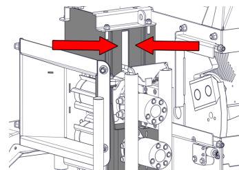
Afbeelding 29 - De walskastsledes smeren
