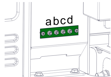
Afbeelding 30 - Smeerpaneel
