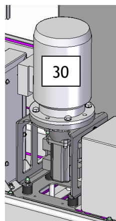
30. Elektromotor
