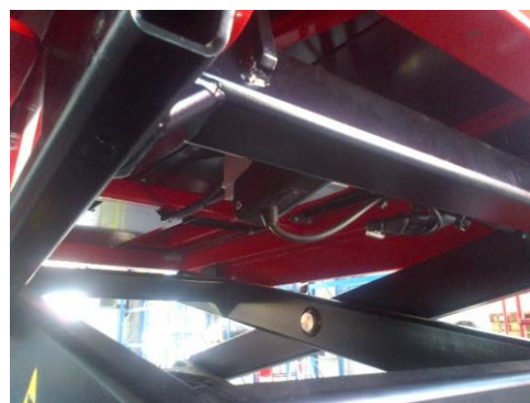
12. Hoeksensor scharen
