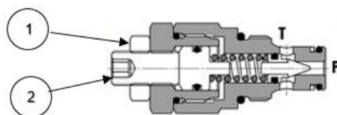
Verklarend schema overdrukventiel
