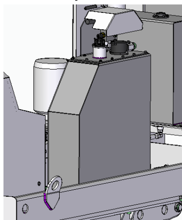
22. Tank hydraulische olie
