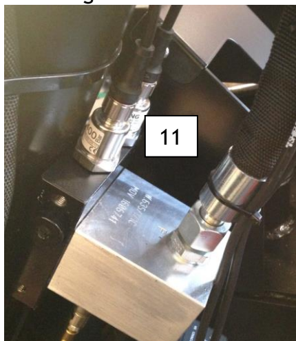
11. Drukomezter voor de controle van de belasting
