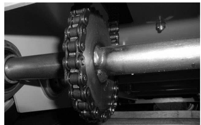
Afbeelding 6.19 Achterzijde voegensnijder, zicht op het kettingwiel van de aandrijvingsas met voortstuwingsketting
