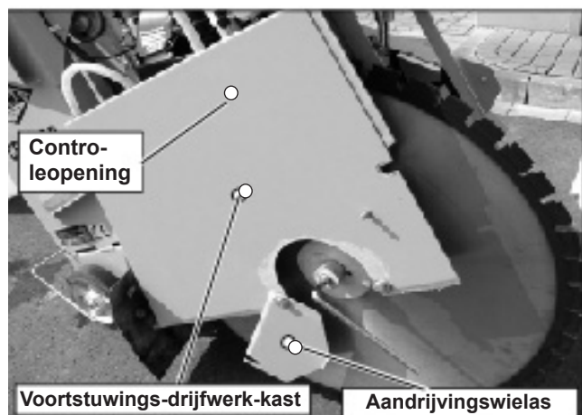
Afbeelding 4.6 CF•2116 D, achterkant
