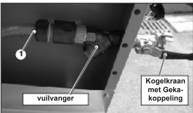
Afbeelding 4.43 CF•2116 D, waterreservoir verwijderd, bladbeveiligings-slang ① aan drukaansluiting gekoppeld
