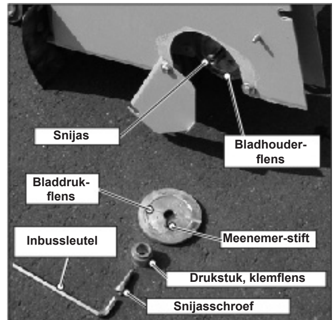
Afbeelding 4.19 CF-2116 D Bladrukflens gedemonteerd
