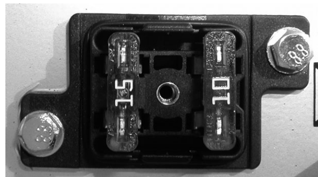
Afbeelding 6.30 CF•2116 D Zekeringenkast (deksel verwijderd)
