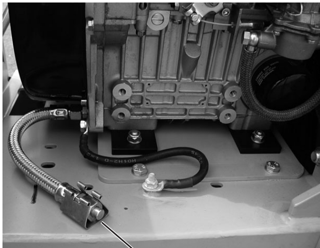
Afbeelding 6.32 CF•2116 D Aftapslang motorolie
