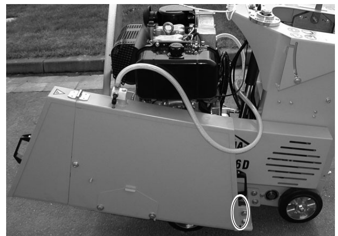
Afbeelding 4.31 Bladbeveiliging aan de linkerkant van de CF-2116 D Standaard gemonteerd
