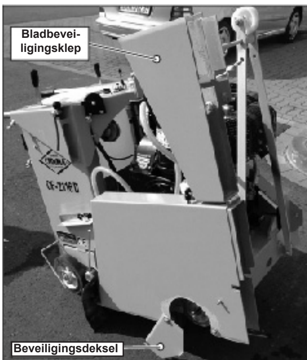
Afbeelding 4.18 CF-2116 D Standaard, bladbeveiliging (rechts gemonteerd), bladbeveiligings-klep geopend en beveiligingsdeksel opgezwinkt
