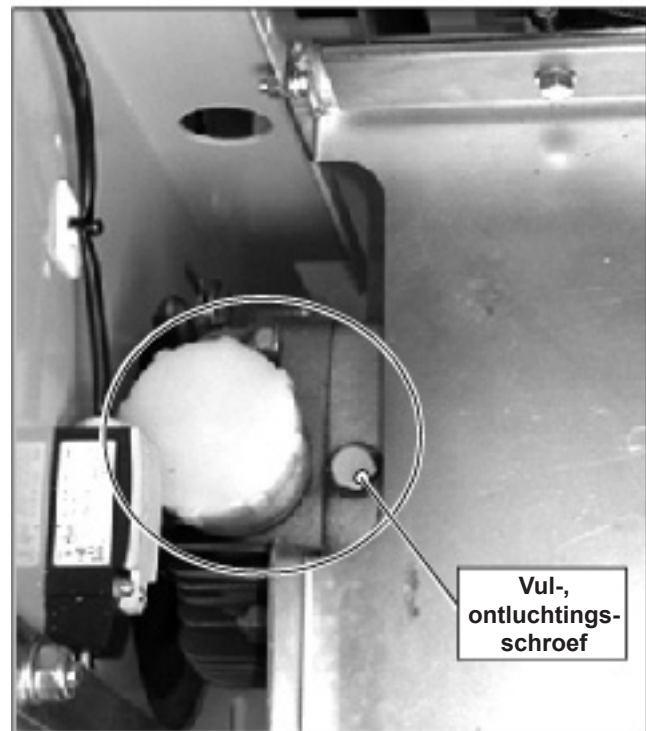
Afbeelding 6.9 CF•2116 D, hydrostatisch voortstuwingsdrijfwerk (waterreservoir verwijderd)
