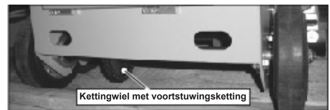
Afbeelding 6.18 Achterkant voegensnijder, zicht op de aandrijvingsas
