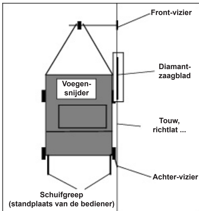
Afbeelding 4.35 CF-2116 D, vizieren uitgelijnd
