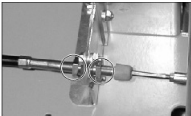
Afbeelding 6.22 CF-2116 D Voortstuwings-bowdenkabel, Contra-, instelmoeren aan behuizing voortstuwingsdrijfwerk
