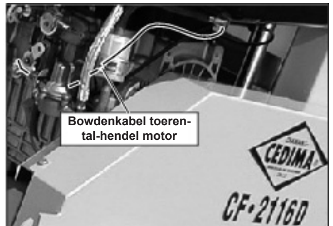
Afbeelding 6.24 CF-2116 D, Bowdenkabel toerentalhendel motor
