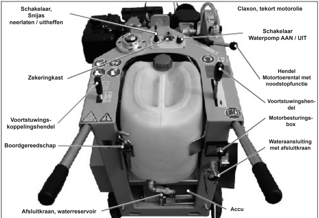
Afbeelding 4.8 Bedieningselementen bij de CF-2116 D, standaard
