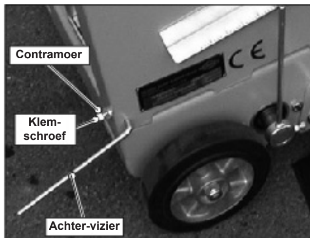
Afbeelding 4.33 CF-2116 D, achternivier (rechts gemonteerd)
