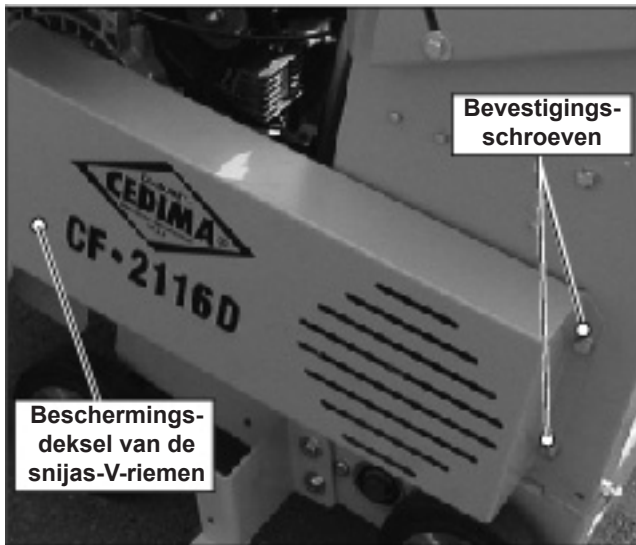
Afbeelding 6.5 CF-2116 D, links
