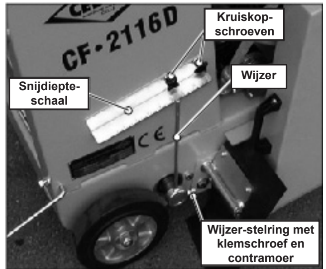
Afbeelding 4.15 snijdiepteweergave
