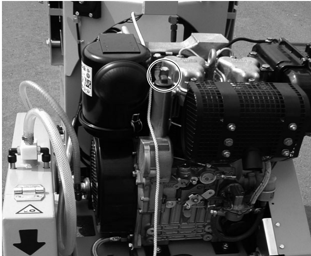
Bild 4.2 CF•2116 D, Motoröl-Einfüllstutzen
