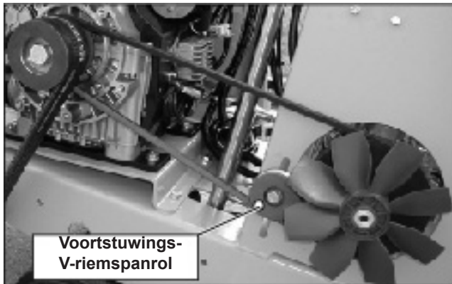
Afbeelding 6.7 CF•2116 D, voortstuwings-V-riem, V-riem-beschermingsdeksel gedemonteerd
