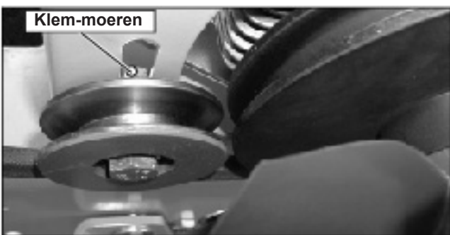
Afbeelding 6.8 CF•2116 D, voortstuwings-V-riem-spanrol, V-riem-spanrol, V-riembeschermingsdeksel gedemonteerd
