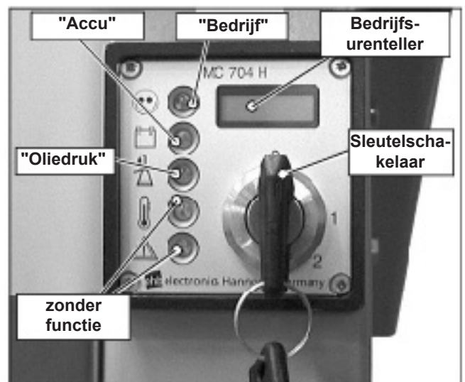
Afbeelding 4.10 motorbesturingsbox met bedrijfsurenteller
