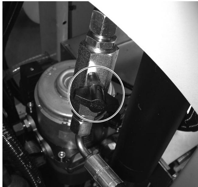
Afbeelding 4.16 smoorklep met borgmoer voor het instellen van de neerlaatsnelheid van de snijas (linker bovenaanzicht op de voegensnijder-montagekast)
