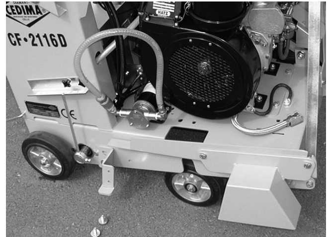
Afbeelding 4.29 Klemschijven- (bladhouderflens-) beveiliging aan de rechter zijde van de CF-2116 D gemonteerd
