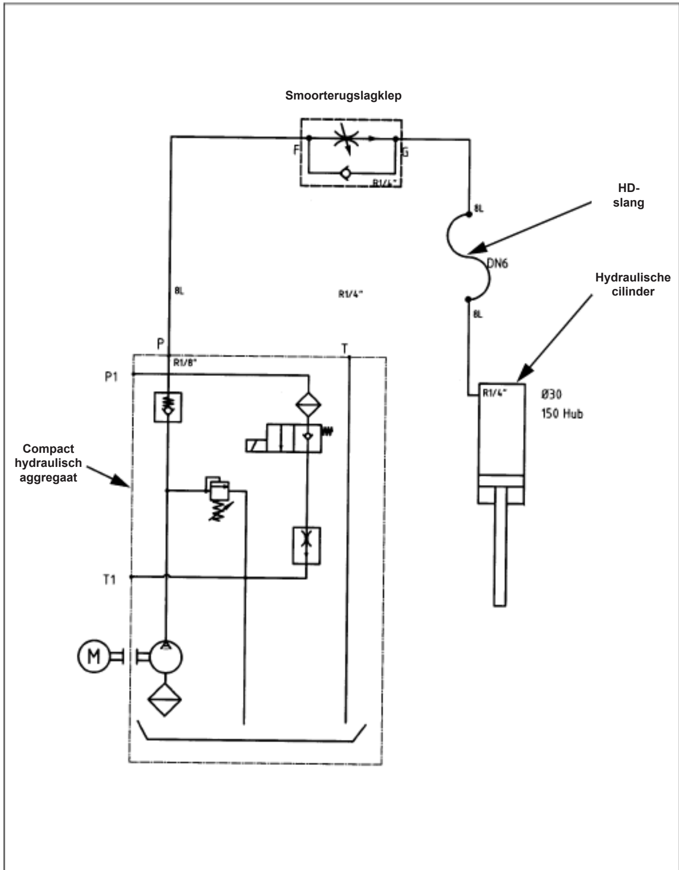
Afbeelding 9.1 CF•2116 D Elektrisch schema
