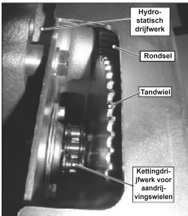
Afbeelding 6.16 CF•2116 D Waterreservoirconsole gede-monteerd, zicht op de behuizing van de voortstuwings-tandwielkast
