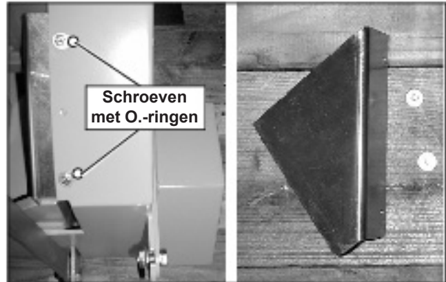
Afbeelding 6.1 Afdekplaat vooraan aan de V-riembescherming
