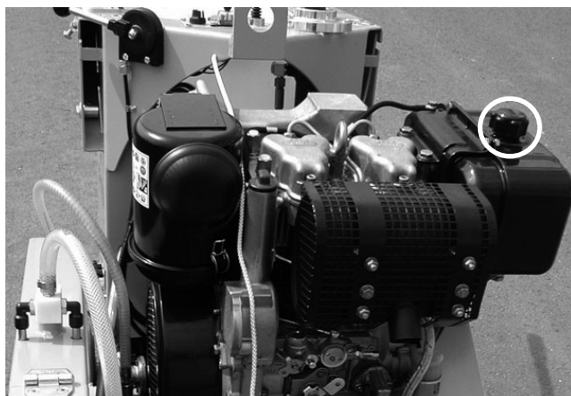
Afbeelding 4.3 CF•2116 D, brandstoftank (tankdeksel)
