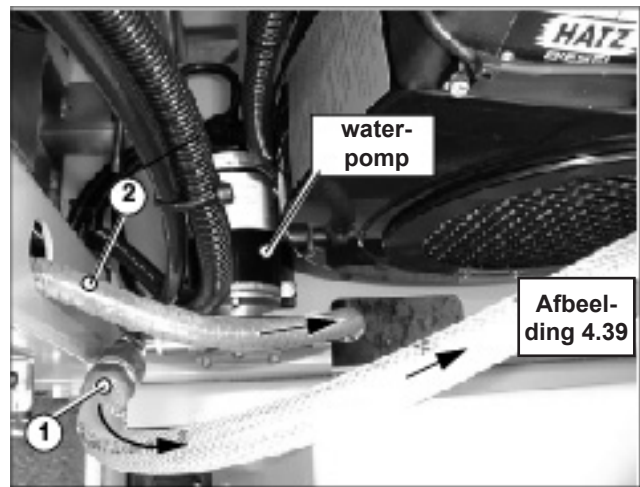
Afbeelding 4.38 CF•2116 D, Bladbeschermings-slang ① aan de Drukaansluiting van de waterpomp aangekoppeld, zuig-slang ② geleid naar waterreservoir
